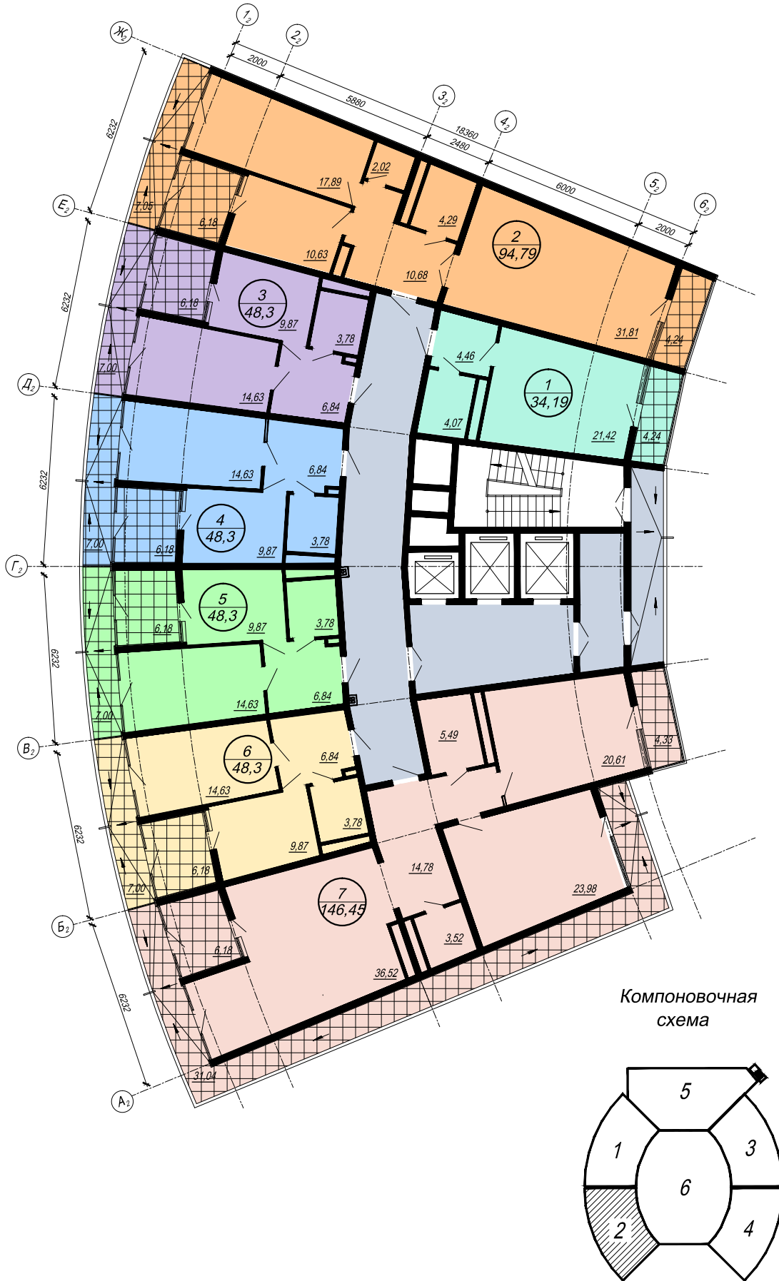
План 4 этажа. Секция 2.
