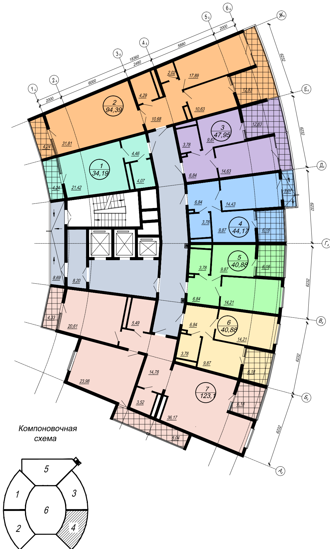
План 13 этажа. Секция 4.
