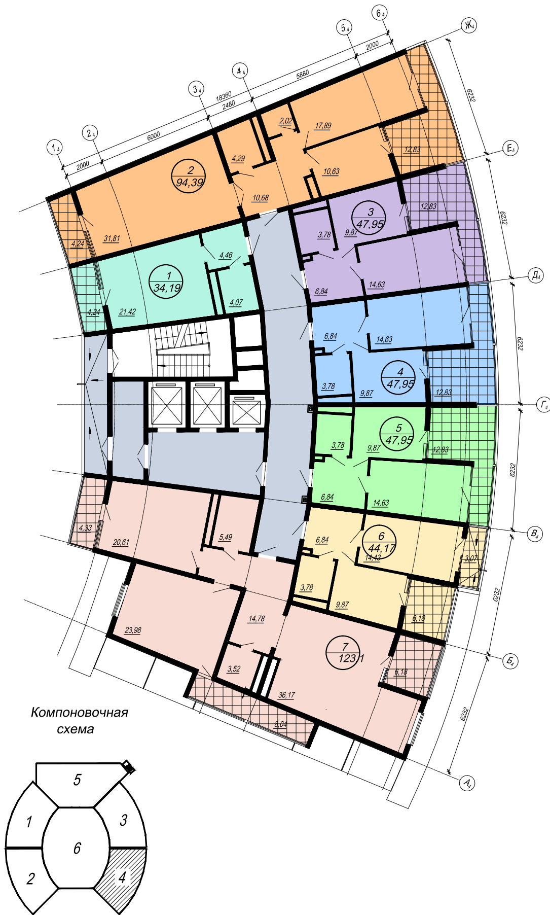
План 8 этажа. Секция 4.
